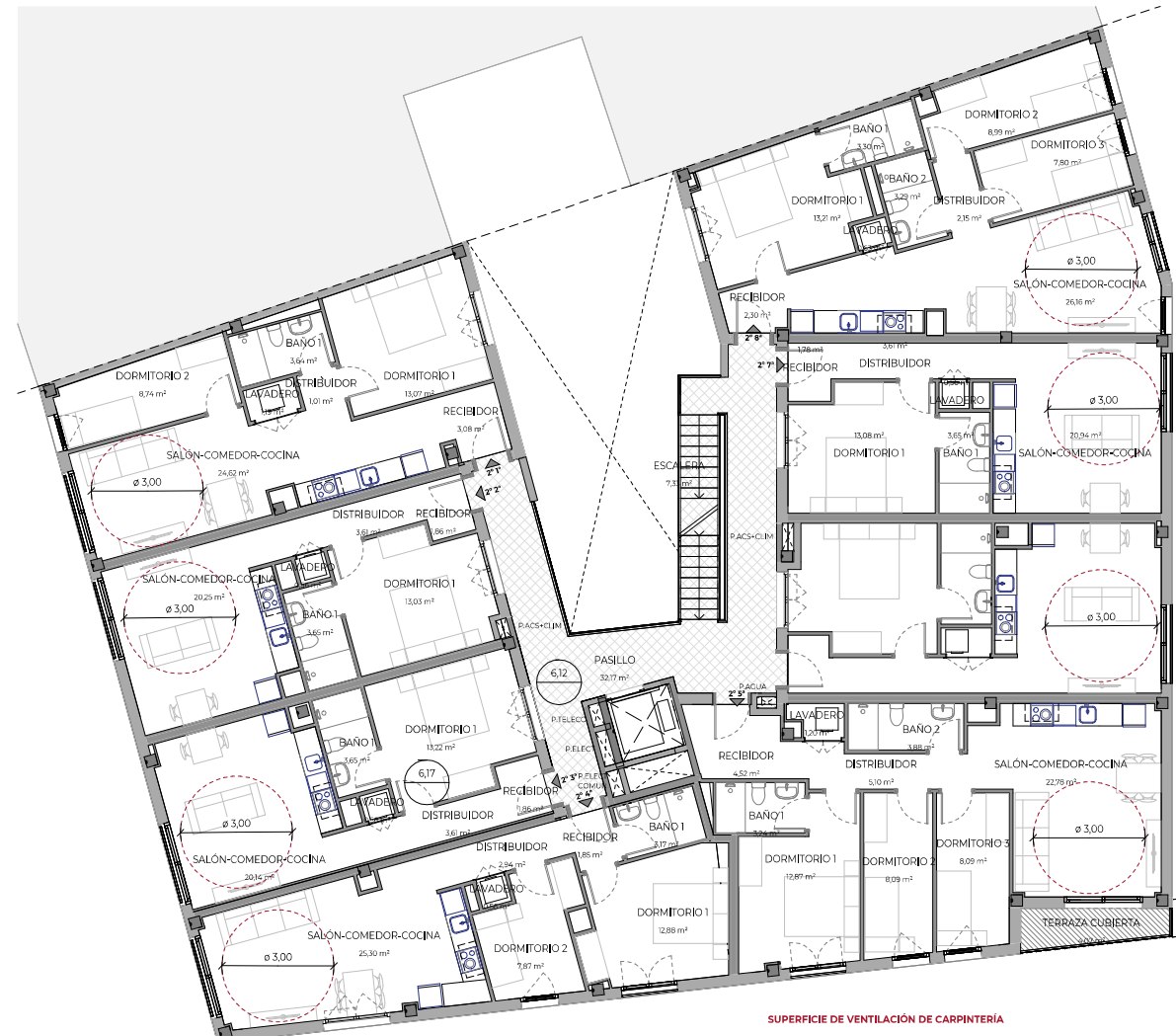
PLANTA TIPO 1:100
