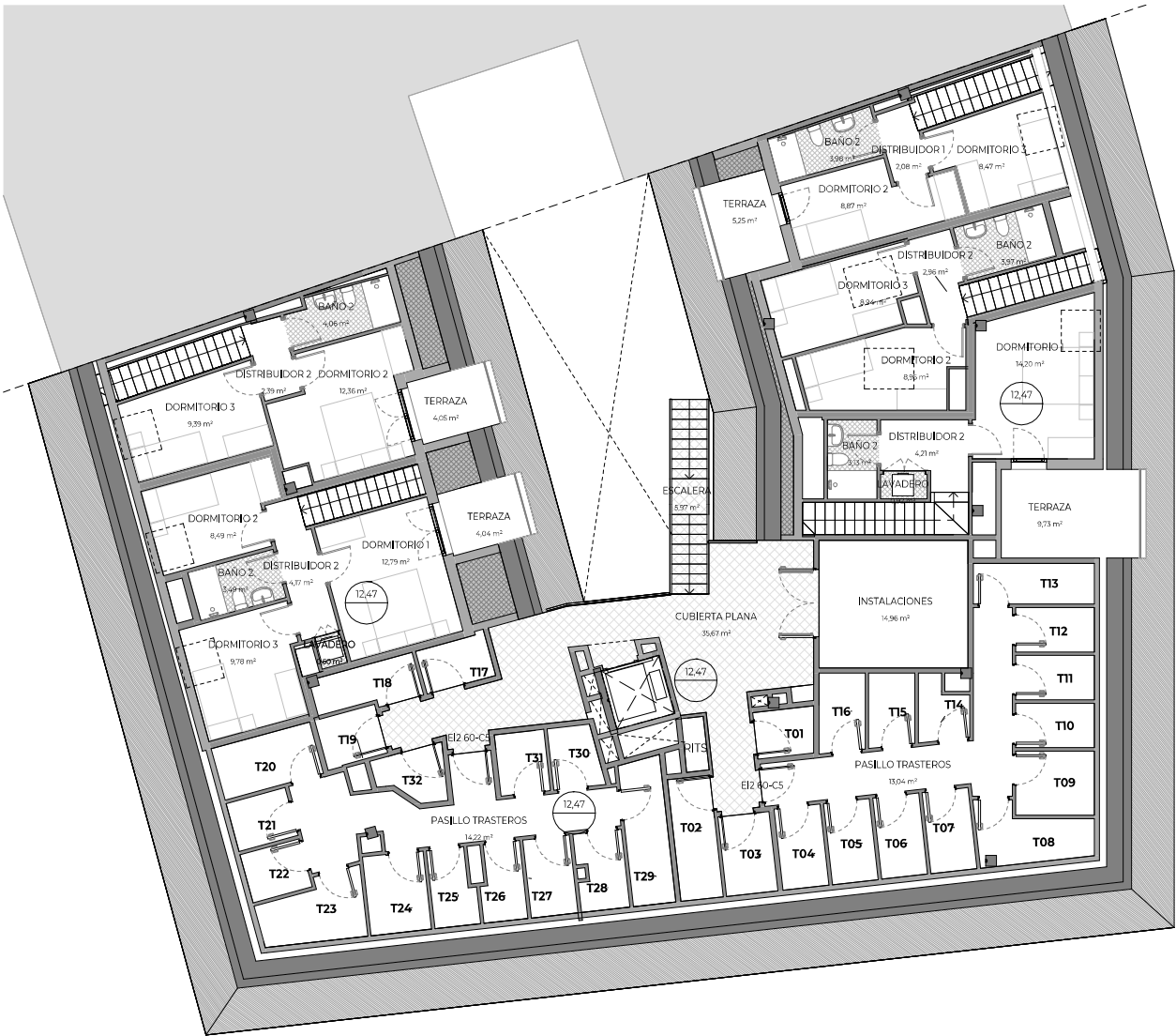
PLANTA BAJOCUBIERTA 1:100
